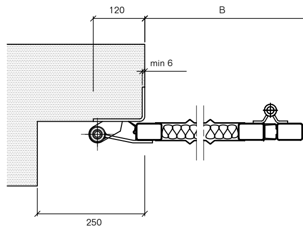
Þröskuldsvinkill Gildir um hurð sem oppnast út.
