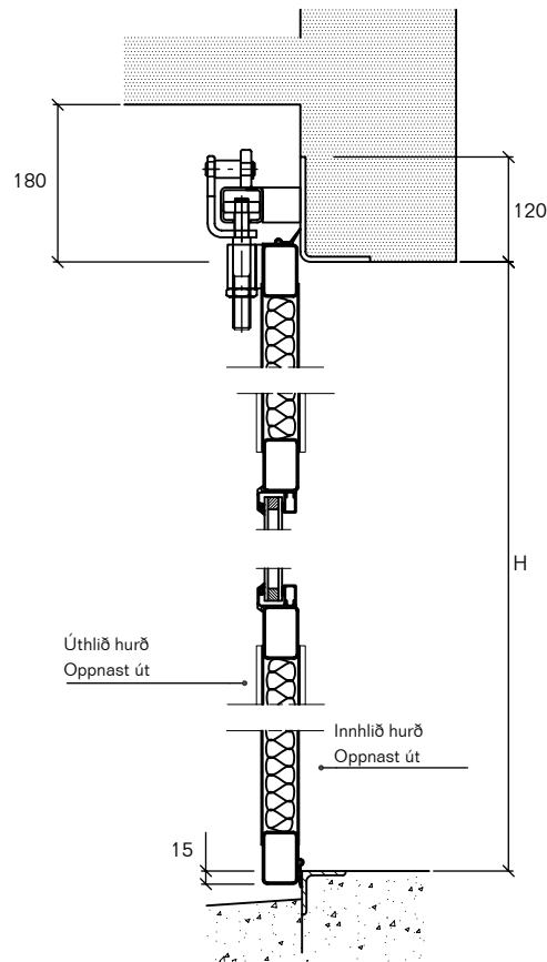
Þröskuldsvinkill Gildir um hurð sem oppnast út.
