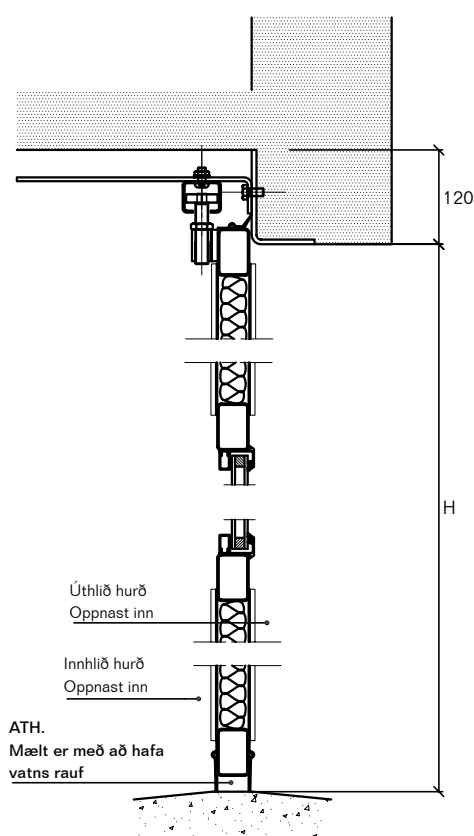
Stýribraut Hurð að 4,5 m á breidd
