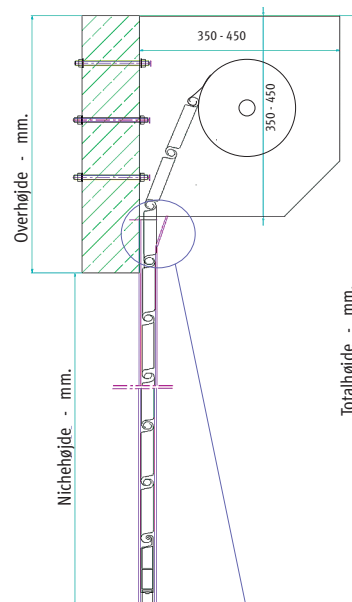
Lodret snit
