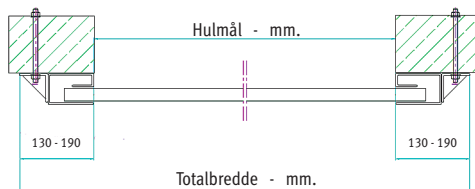
Vandret snit
