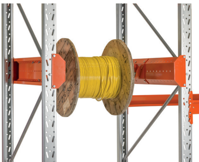
Keflaslá - með sjálflæsandi öxli. Stillanleg festing fyrir kefli. Í 950 og 1350 mm bil.
