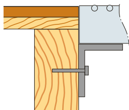
Alt 1. Kåbe Hyllprofil 25RH
