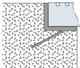
Alt 2. Kåbe Ingjutningsprofil 25RI
