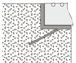
Alt 3. Kåbe ingjutningsprofil 25RI
