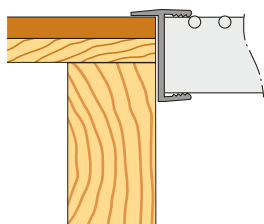
Alt 1. Kåbe Hängprofil
